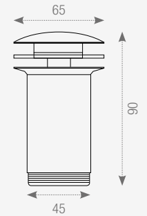
VALVULA ONE TOUCH NEGRO MATE
